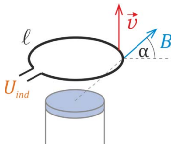
Obr. 5. Indukované napětí pro závit v obecnější poloze je U = v B l \cos \alpha .
