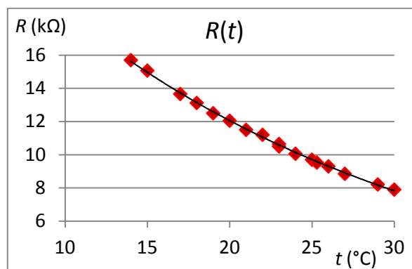
Obr. 1. Perličkový termistor 10 k \Omega a změřená závislost jeho odporu na teplotě
