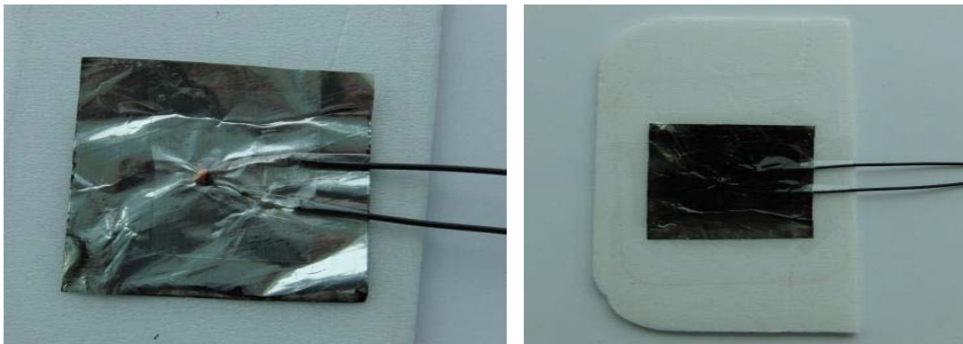
Obr. 2. Konstrukce detektoru tepelného záření: termistor přilepený na alobal, lesklou stranou položený na kousek polystyrénu; vnější strana alobalu je začerněna.
